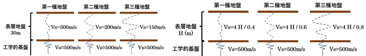
図 1 地盤モデル 1
